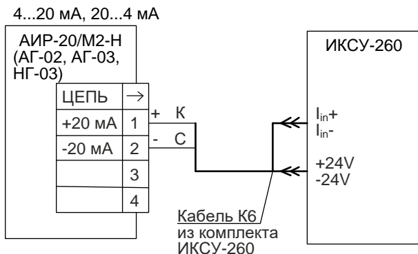
Рисунок 3.1 – Схема электрическая подключений. Вариант с полярностью подключения питания «K1+»
