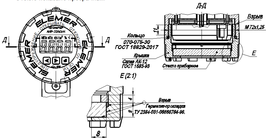
Рисунок А.4 – Чертеж средств взрывозащиты
