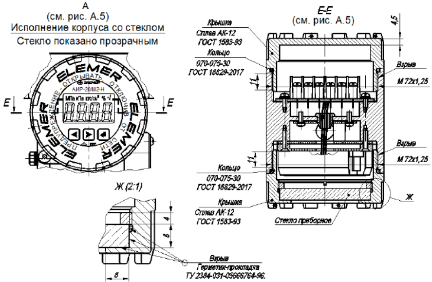
Рисунок А.7 – Чертеж средств взрывозащиты
