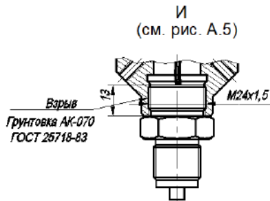
Рисунок А.8 – Чертеж средств взрывозащиты
