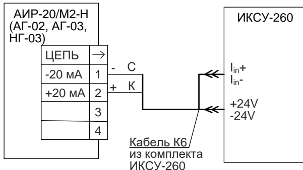
Рисунок 3.4 – Схема электрическая подключений. Вариант с полярностью подключения питания «K1-»
